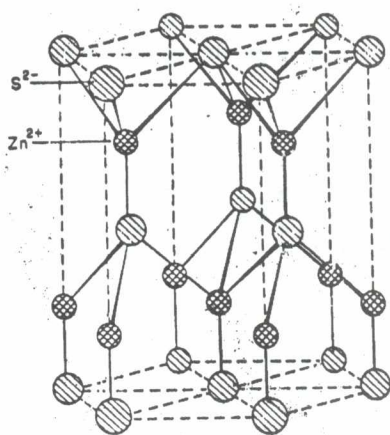
Fig 3.1: Wurtzite (ZnS) structure
