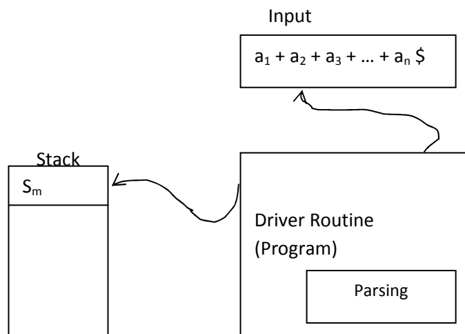
Fig. 2: LR Parser
