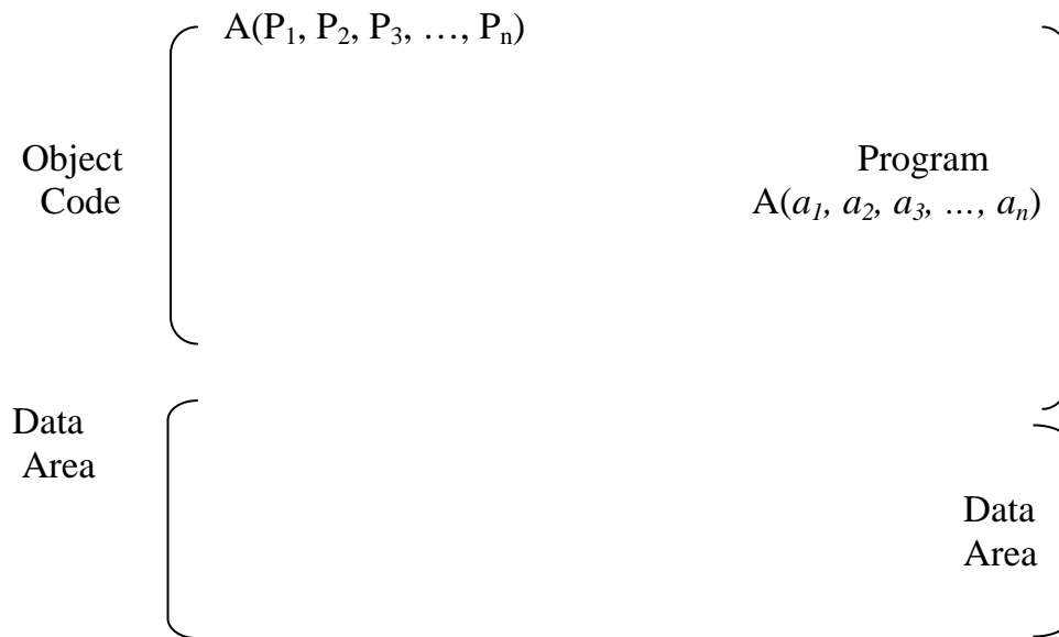
Fig. 4: Actual-Formal Parameter Correspondence
